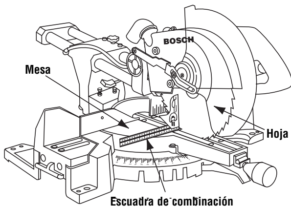
Figura 5. Hoja en ángulo recto con la mesa
