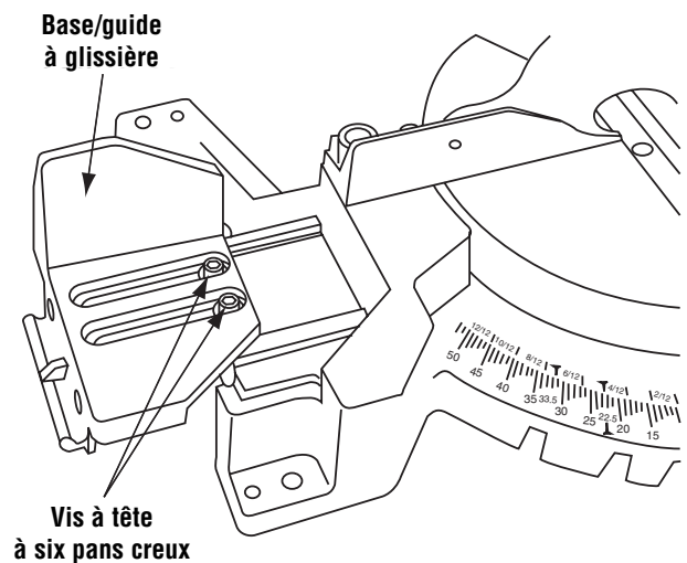
Figure 26. Base/guide à glissière
