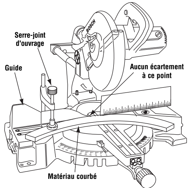
Figure 36. Matériau courbé
