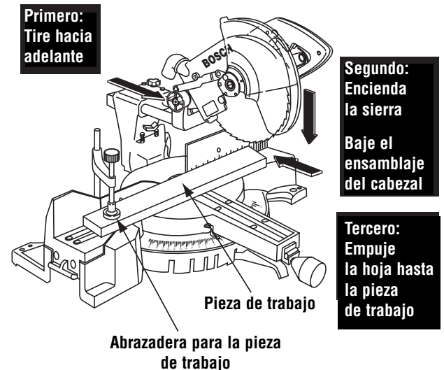
Figura 28. Corte deslizante
