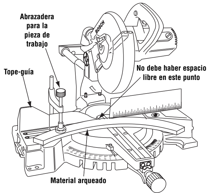
Figura 36. Material arqueado
