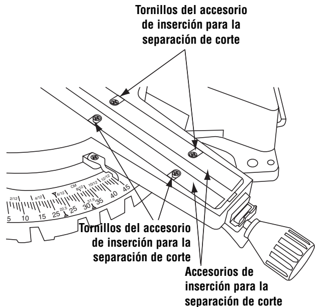
Figura 13. Accesorio de inserción para la separación de corte
