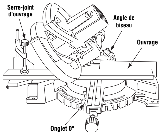
Figure 30. Coupe en biseau
