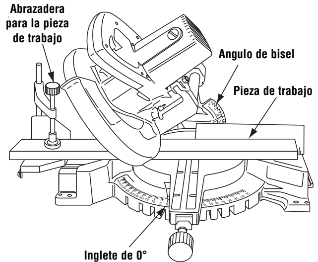
Figura 30. Corte en bisel
