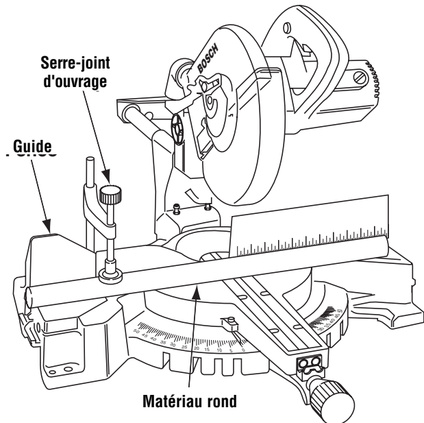
Figure 37. Matériau rond
