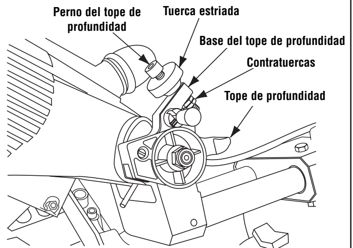
Figura 14. Ajuste del tope de profundidad
