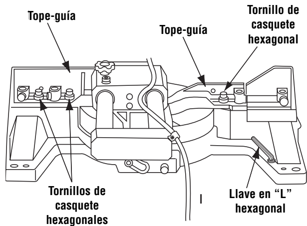
Figura 11. Ajuste del tope-guía
