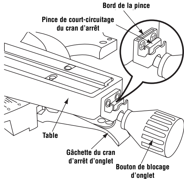
Figure 25. Court-circuitage du cran d'arrêt
