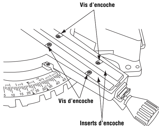
Figure 13. Insert d'encoche
